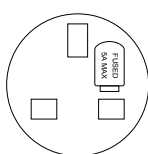
2P+E socket
