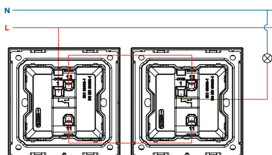
○5 1G 2W switch
