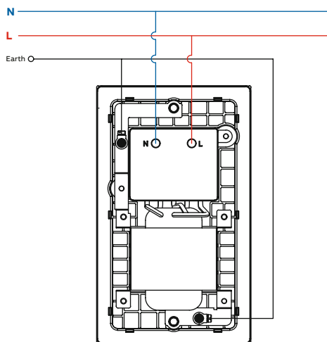
O16 Shaver unit
