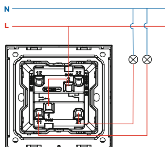
○2 2G 1W switch
