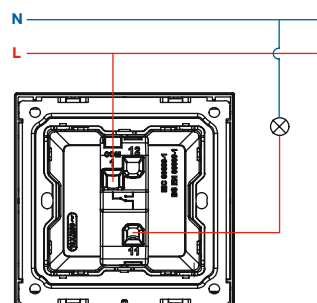
○1 1G 1W switch
