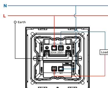
○9 1G 1W switch 20AX DP
