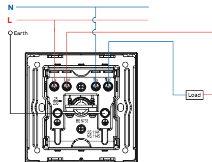
O15 Flex outlet 25A
