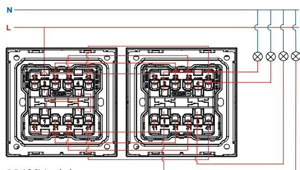
○8 4G 2W switch
