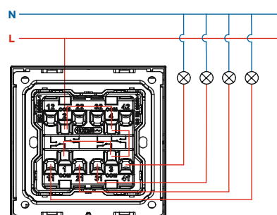
○4 4G 1W switch
