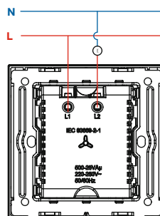
O35 Fan regulator
