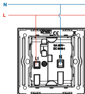
O21 2G 10A Euro-American Switch Socket
