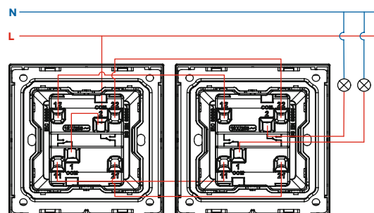
○6 2G 2W switch
