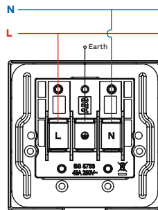
O14 Flex outlet 45A
