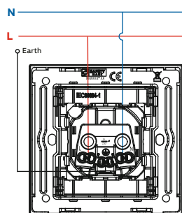
O23 1G 16A SCHUKO Socket
